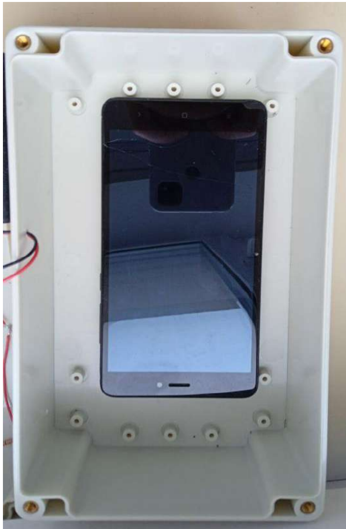
Рисунок 4.13 — Макет пристрою з телефоном всередині
