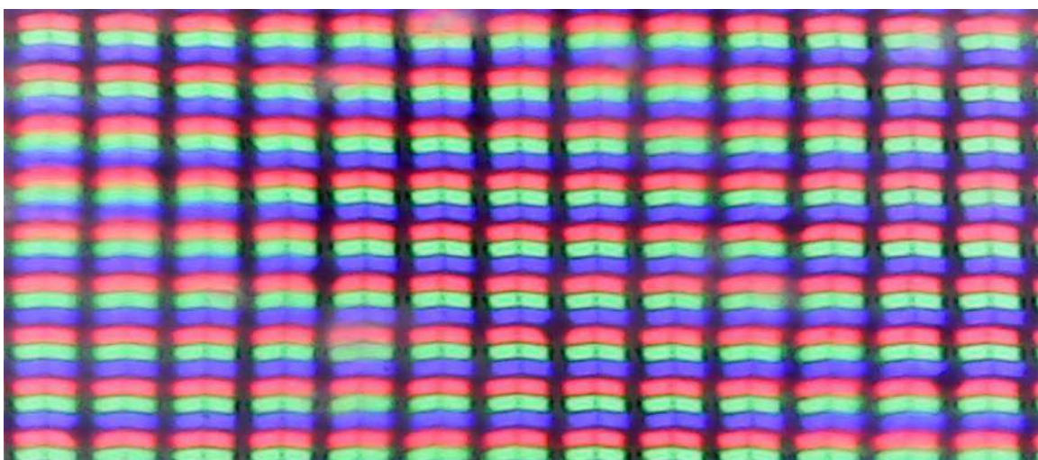
Рисунок 4.35 — Вигляд OLED дисплею після дії УФ-опромінення потужністю 6 Вт та тривалістю опромінення 10 хвилин
