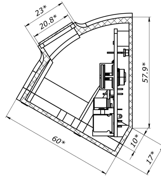
SECTION A-A SCALE 4 : 3
